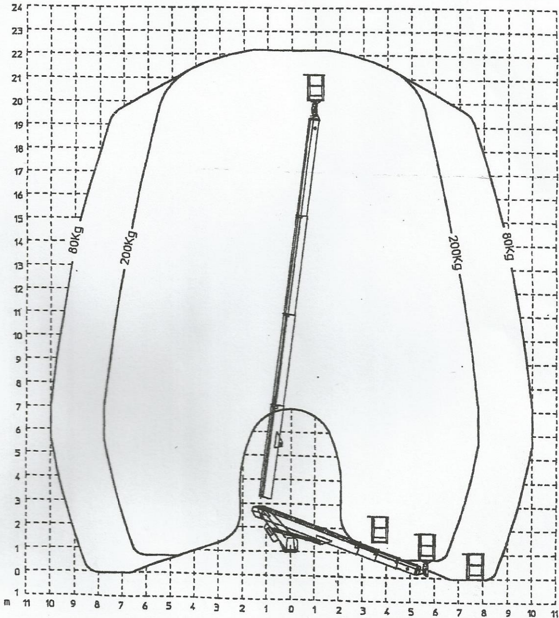
MERCEDES 308 D - 3550 mm
