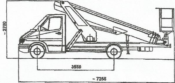
MERCEDES 308 D - 3550 mm
